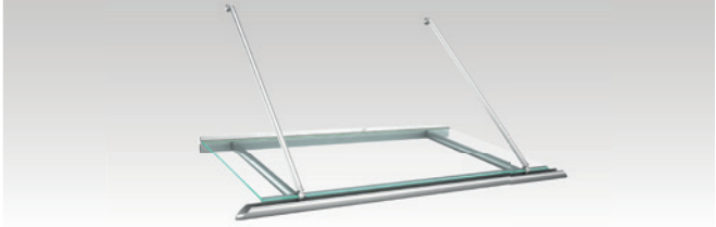
CALYPSO I VSG Modellgröße*: 1.600 x 950 mm Füllung: VSG-Verglasung Standardfarbe: RAL: 7016 matt; 9007 matt; DB703 matt; 9016 weiß
