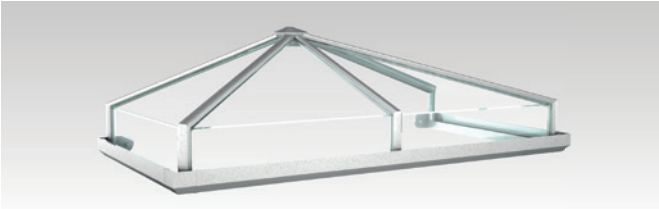
KRISTALL I ACRYL Modellgröße*: 1.800 x 925 mm Füllung: Acryl-Verglasung Standardfarbe: RAL: 7016 matt; 9007 matt; DB703 matt; 9016 weiß
