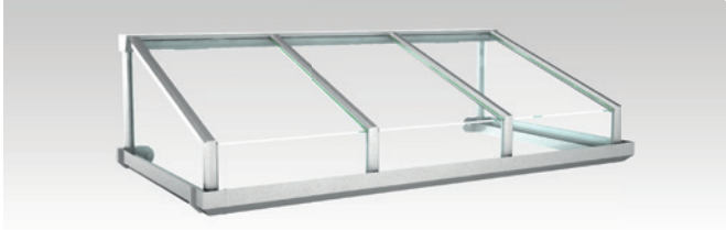
MARIN ACRYL Modellgröße*: 1.600 x 1.000 mm Füllung: Acryl-Verglasung seitl. geschlossen Standardfarbe: RAL: 7016 matt; 9007 matt; DB703 matt; 9016 weiß
