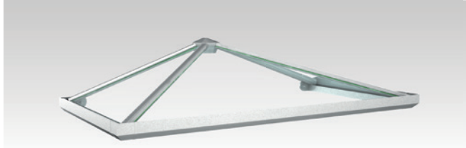
CORALL I VSG Modellgröße*: 2.000 x 1.025 mm Füllung: VSG-Verglasung Standardfarbe: RAL: 7016 matt; 9007 matt; DB703 matt; 9016 weiß
