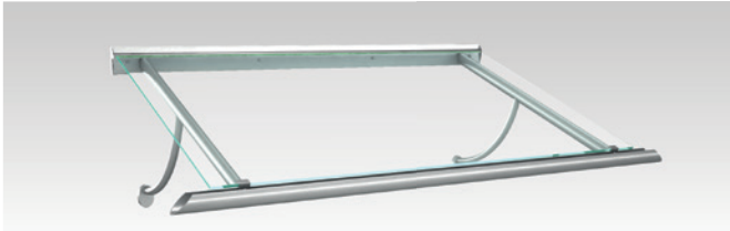
CALYPSO VSG Modellgröße*: 1.600 x 950 mm Füllung: VSG-Verglasung Standardfarbe: RAL: 7016 matt; 9007 matt; DB703 matt; 9016 weiß
